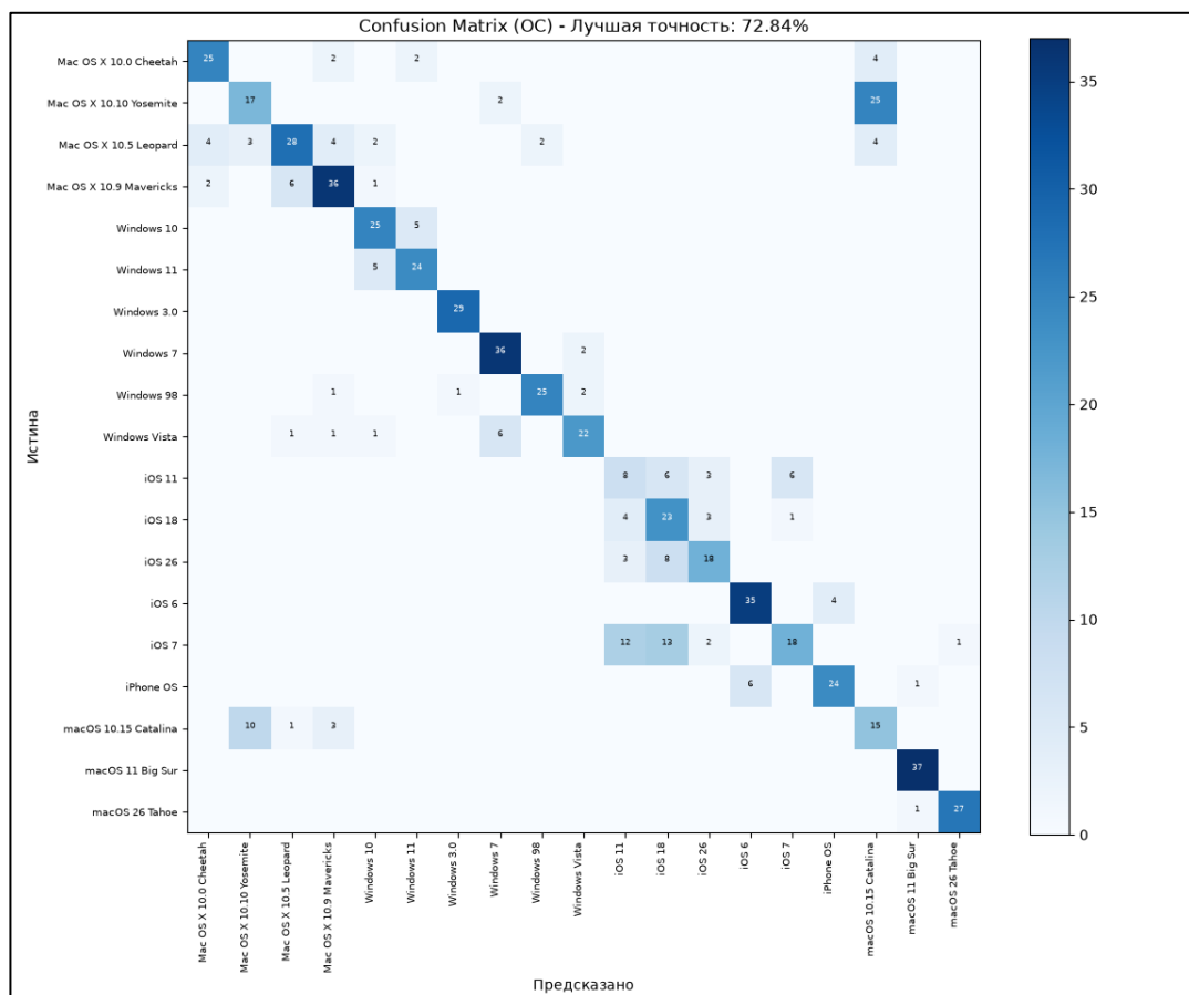
Рисунок 6.12 – матрица неточностей для классификатора ОС
