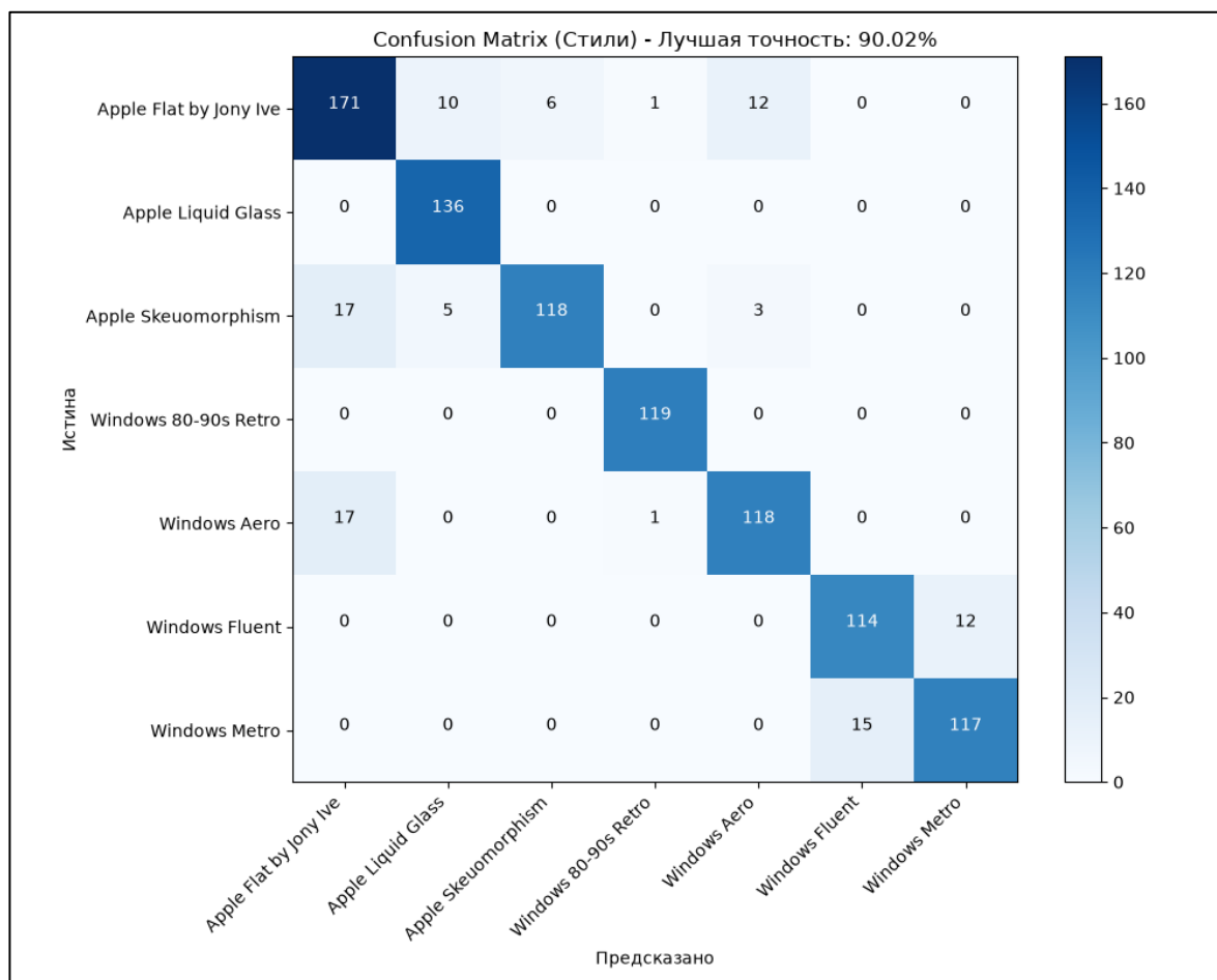
Рисунок 6.8 – матрица неточностей для классификатора стилей
