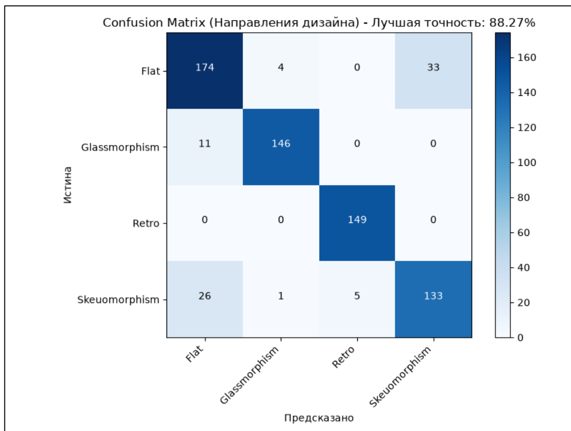
Рисунок 6.4 – матрица неточностей для классификатора направлений дизайна
